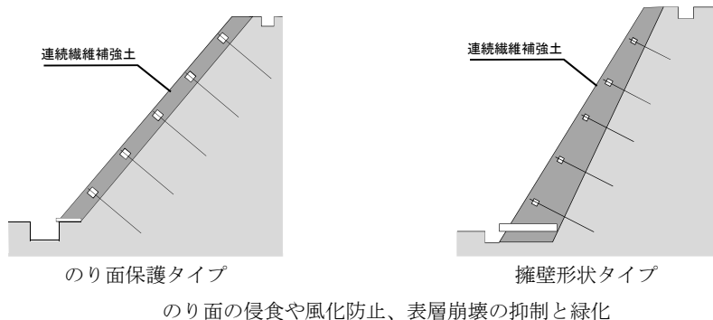
図 1-1 ジオファイバー工法の主な用途例
