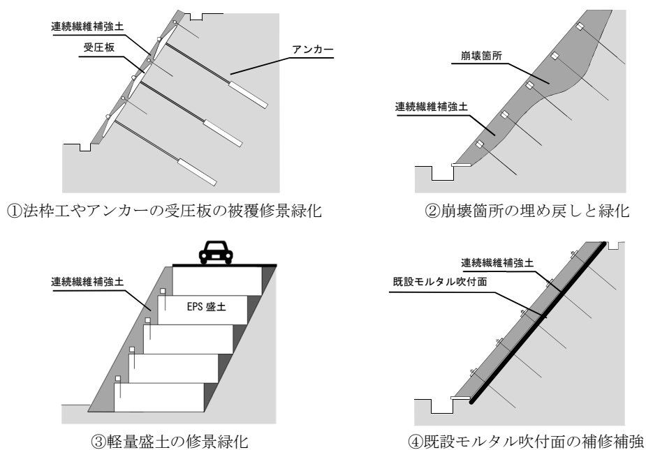
図 1-2 ジオファイバー工法の代表的な用途例
