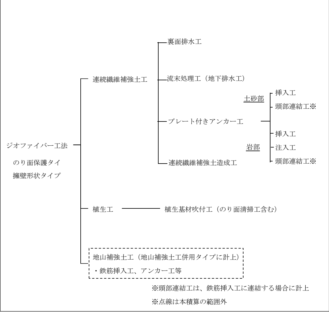
ジオファイバー工法の積算基本構成
