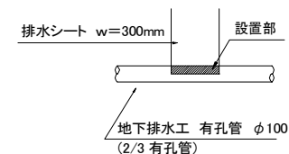
接続部詳細図
