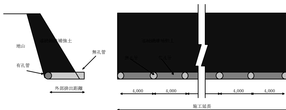
図 5-2 流末処理工
