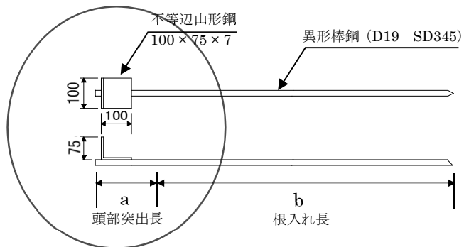
図 2-6 プレート付アンカー
