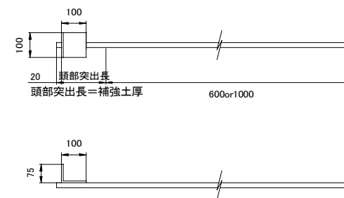
プレート付きアンカー詳細図
