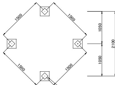
地山補強土工配置図例
