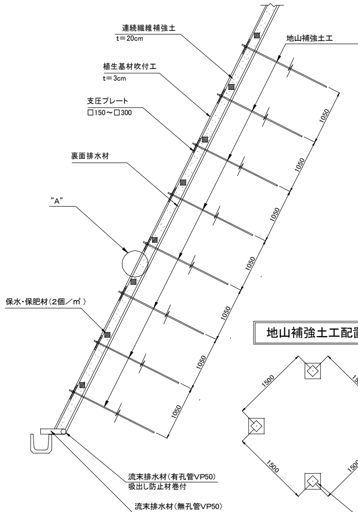
断面図
