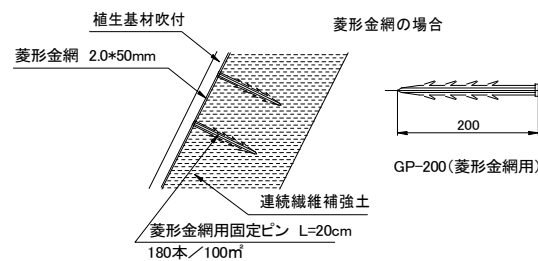
"A"詳細図
