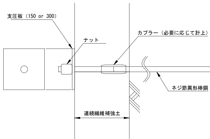
図 2-7 支圧板付きアンカー
