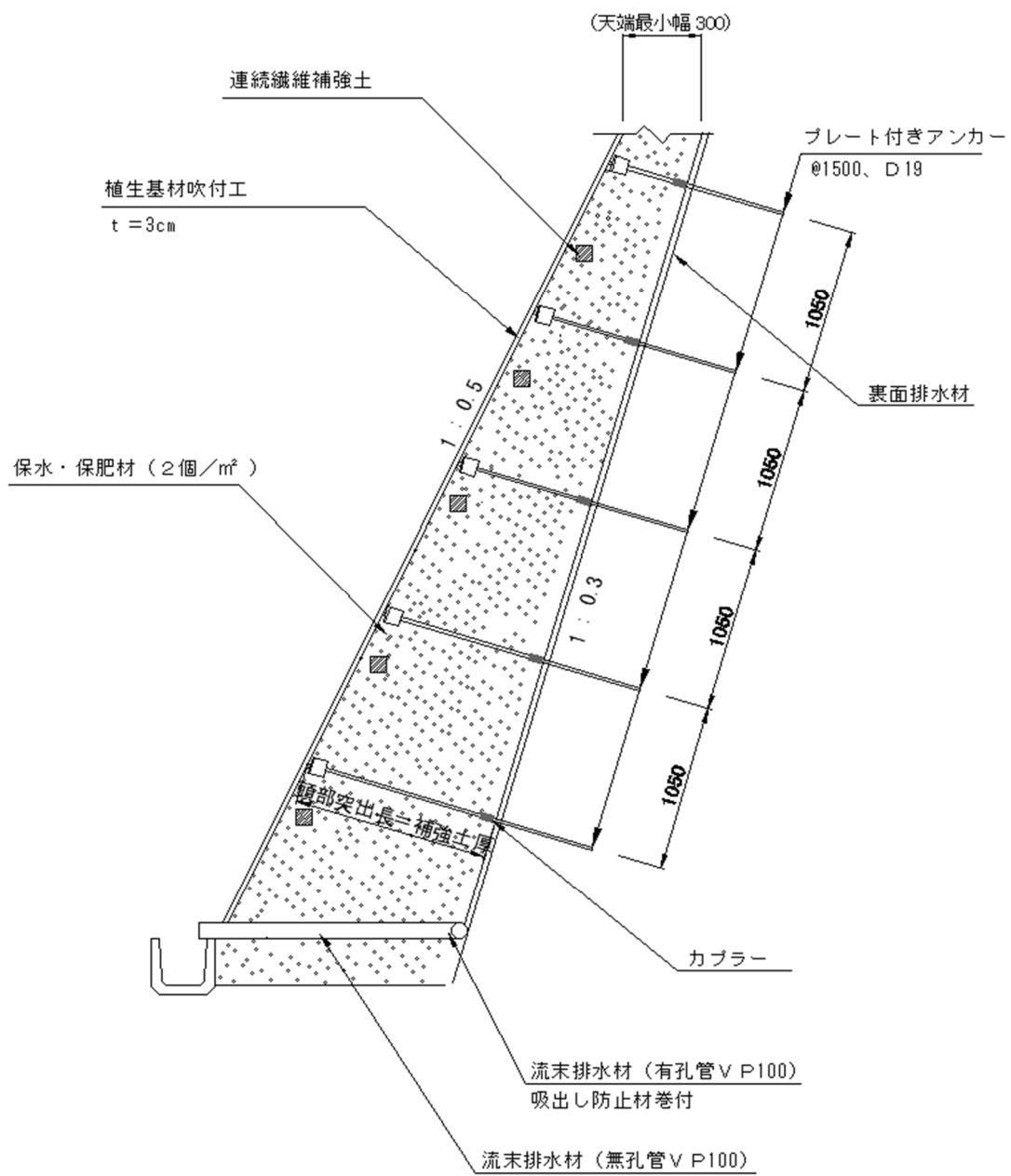
図 2-4 擁壁形状タイプ
