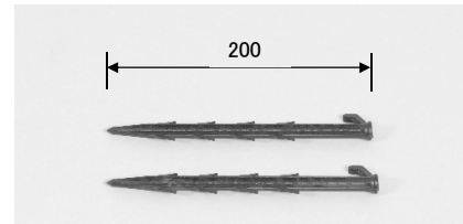
ジオピン(GP-200)
