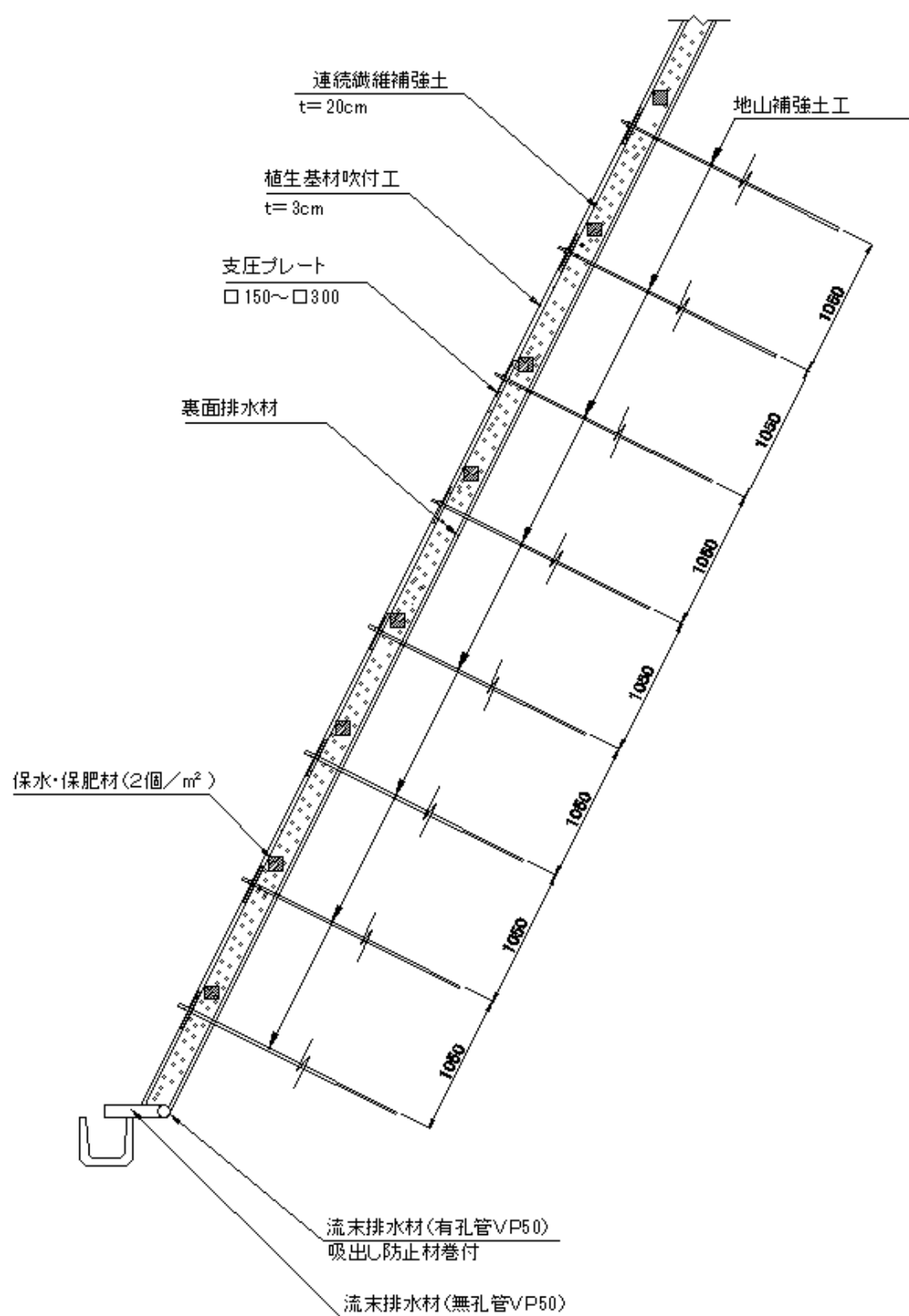
図 2-3 のり面保護タイプ(地山補強土工併用タイプ)
