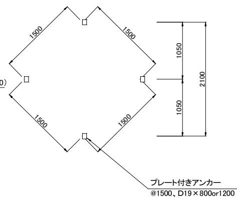
プレート付きアンカー配置図
