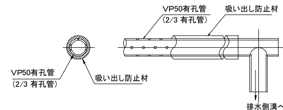
接続部詳細図
