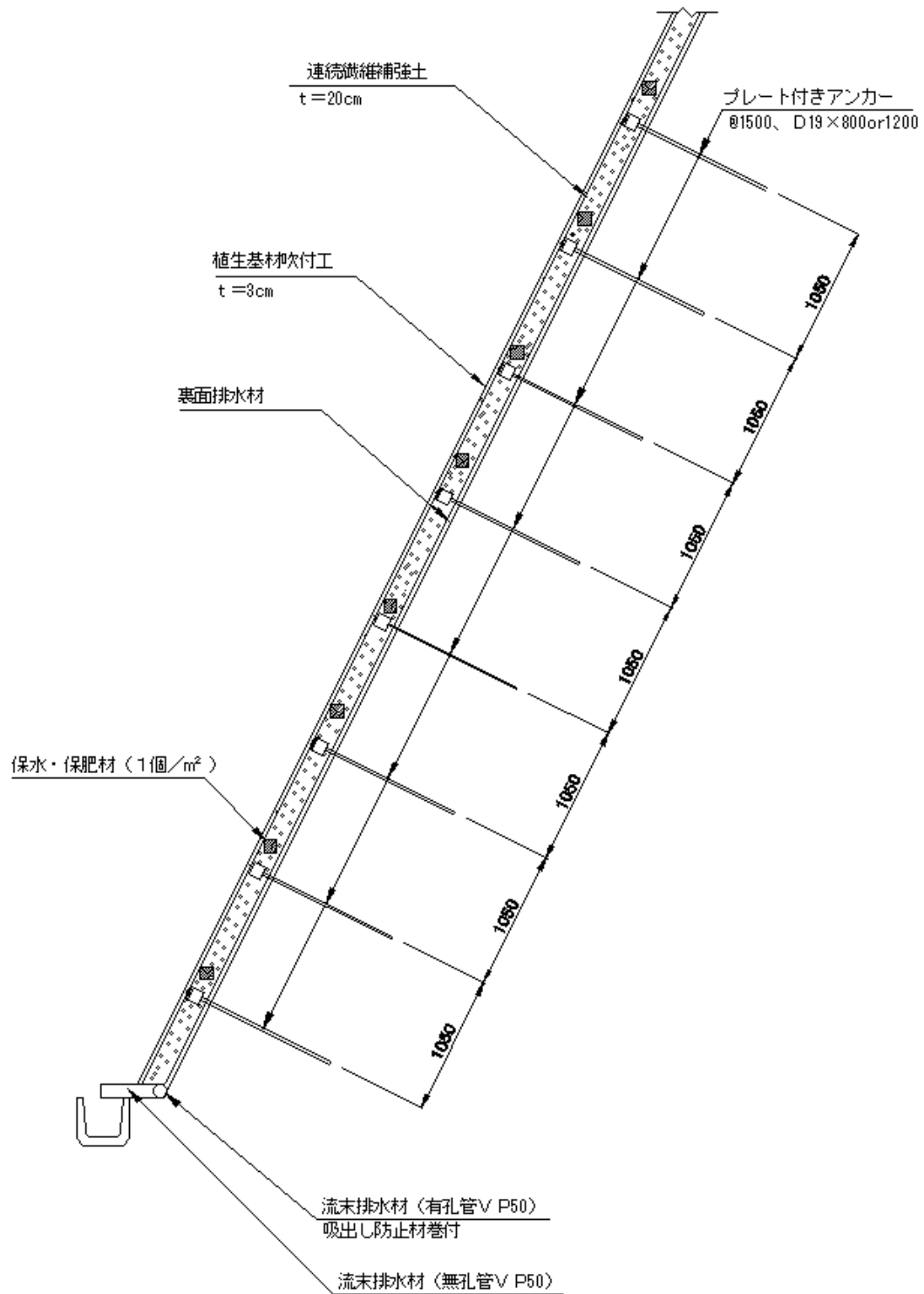
図 2-2 のり面保護タイプ
