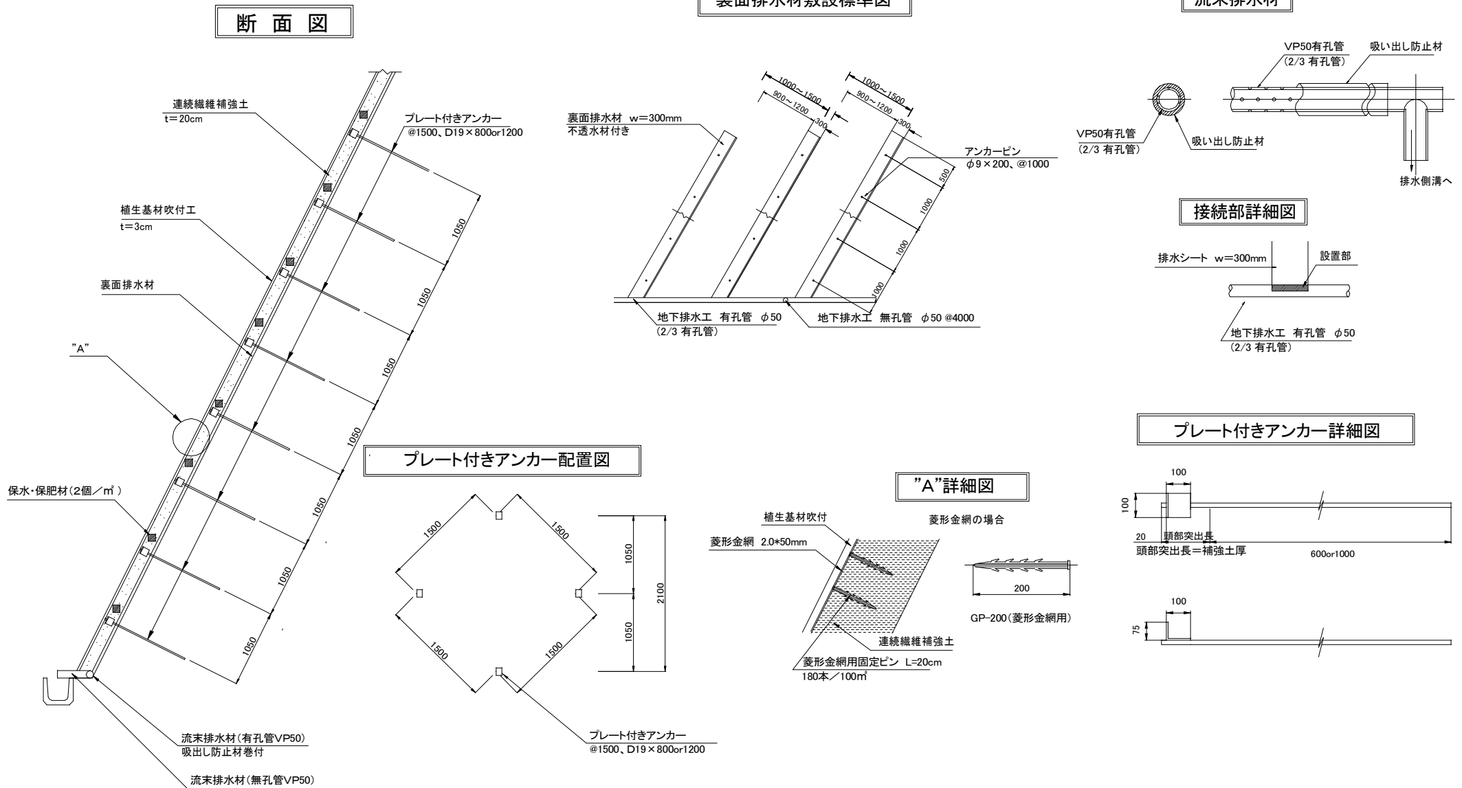
裏面排水材敷設標準図
