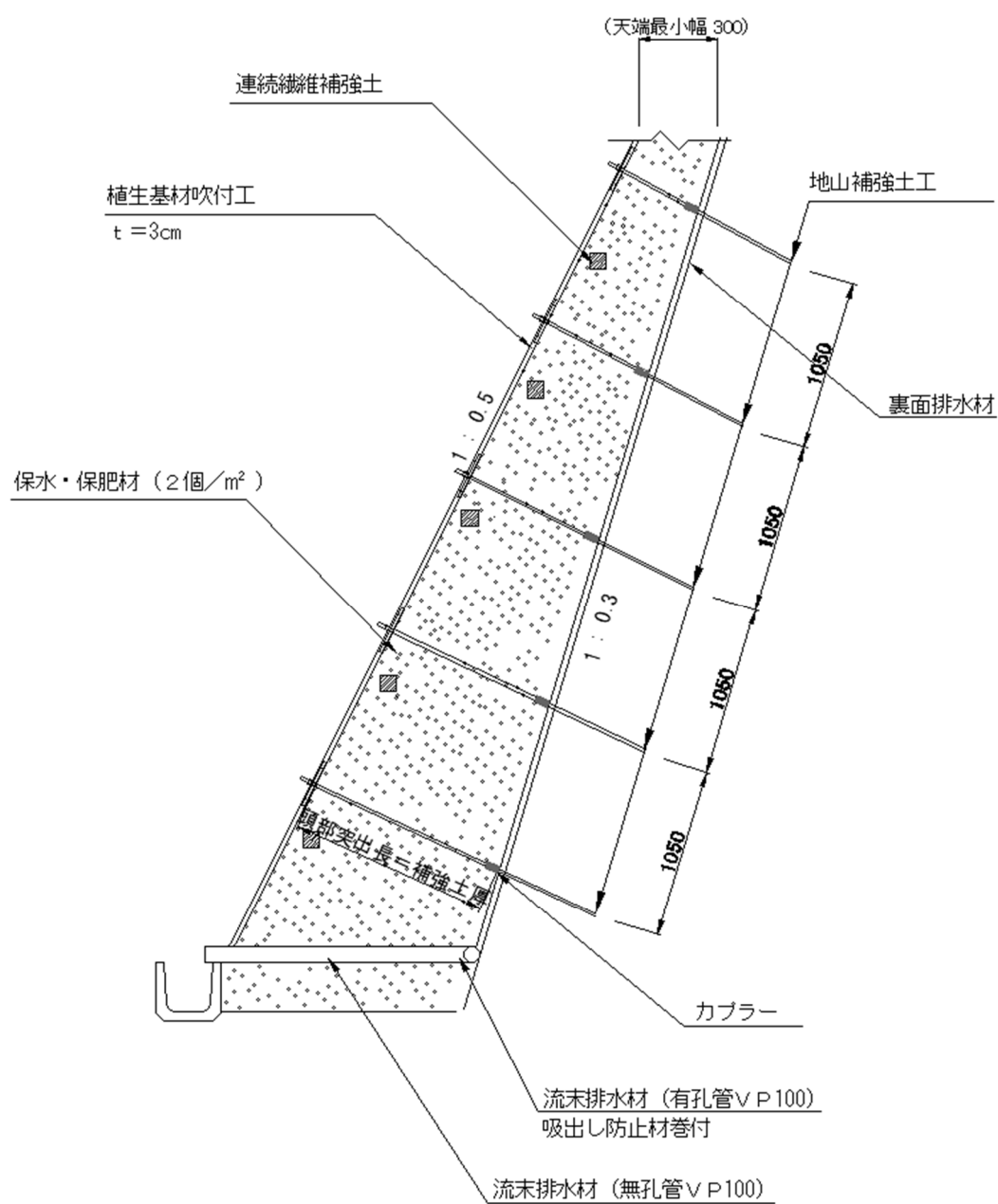
図 2-5 擁壁形状タイプ(地山補強土工併用タイプ)
